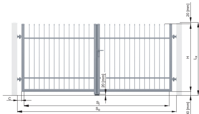
Obr. 9. Rozměry potřebné pro správný výběr a montáž dvoukřídlé brány - pohled z pozemku.
