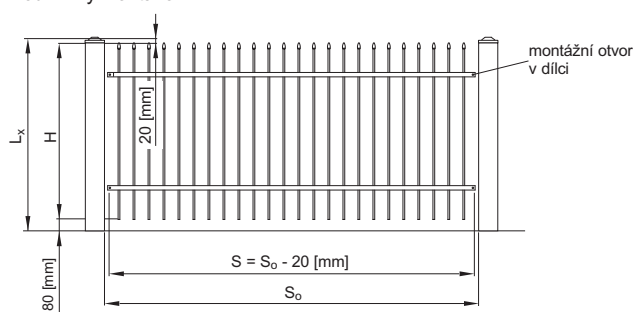
Obr. 2. Montážní rozměry potřebné pro správný výběr a montáž plotového dílce.
