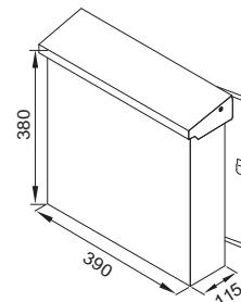
Obr. 7. Poštovní schránka BOX 2.
