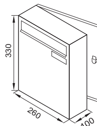
Obr. 6. Poštovní schránka BOX 1.
