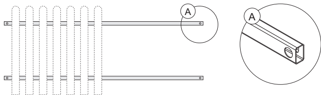
Obr. 8. Vodorovné příčky pro montáž individuální výplně.
